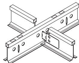
Epaulement de l'entretoise sur le porteur.
