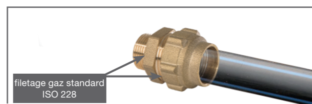
L'étanchéité se fait par joint torique gros diamètre
