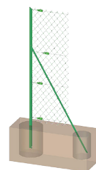
Piquet cornière de départ avec jambe de force, tendeurs, fil de tension et grillage Simple Torsion
