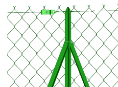
Piquet Té intermédiaire avec jambes de force
