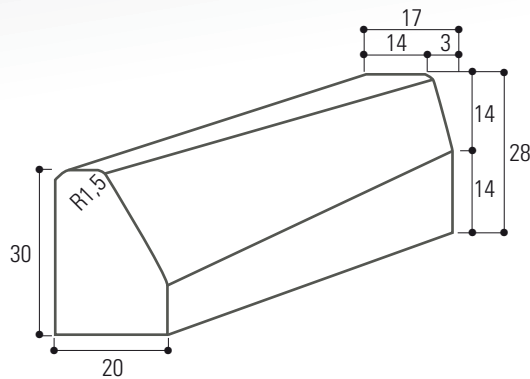
Raccord T3/quai bus droite et gauche
