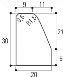
Bordure quai bus
