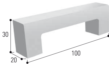
Bordure 20 x 30 avaloir traversant
