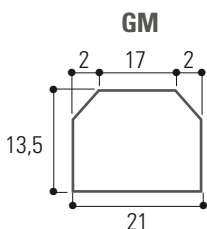
Bordure délimitation piste cyclable
