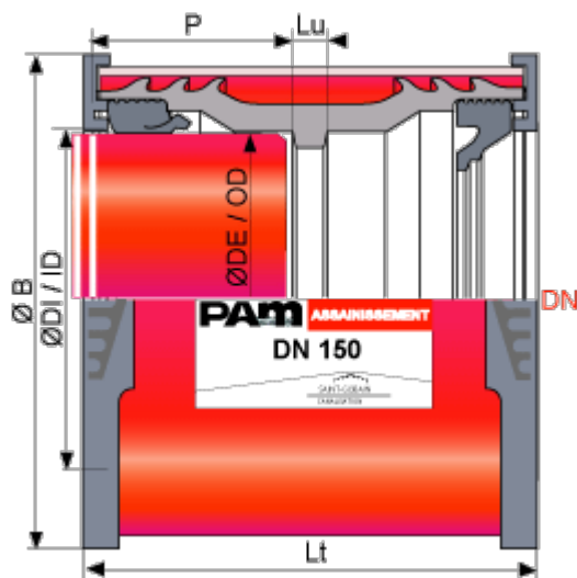
[1] DN 150 et 200
