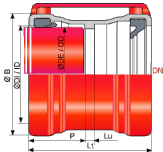
[2] DN 250 et 300
