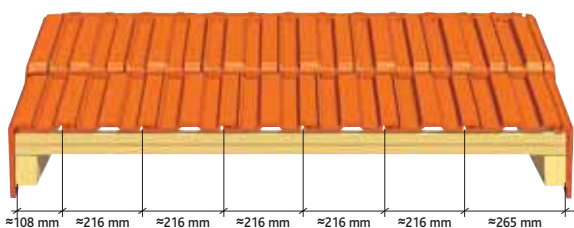
Pose avec rives individuelles
