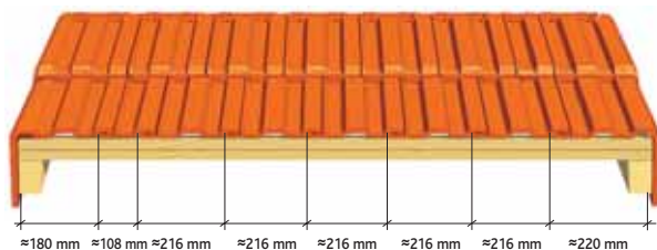
Pose avec rives individuelles
